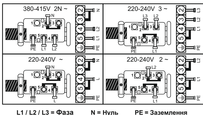
L1 / L2 / L3 = Фаза N = Нуль PE = Заземлення
